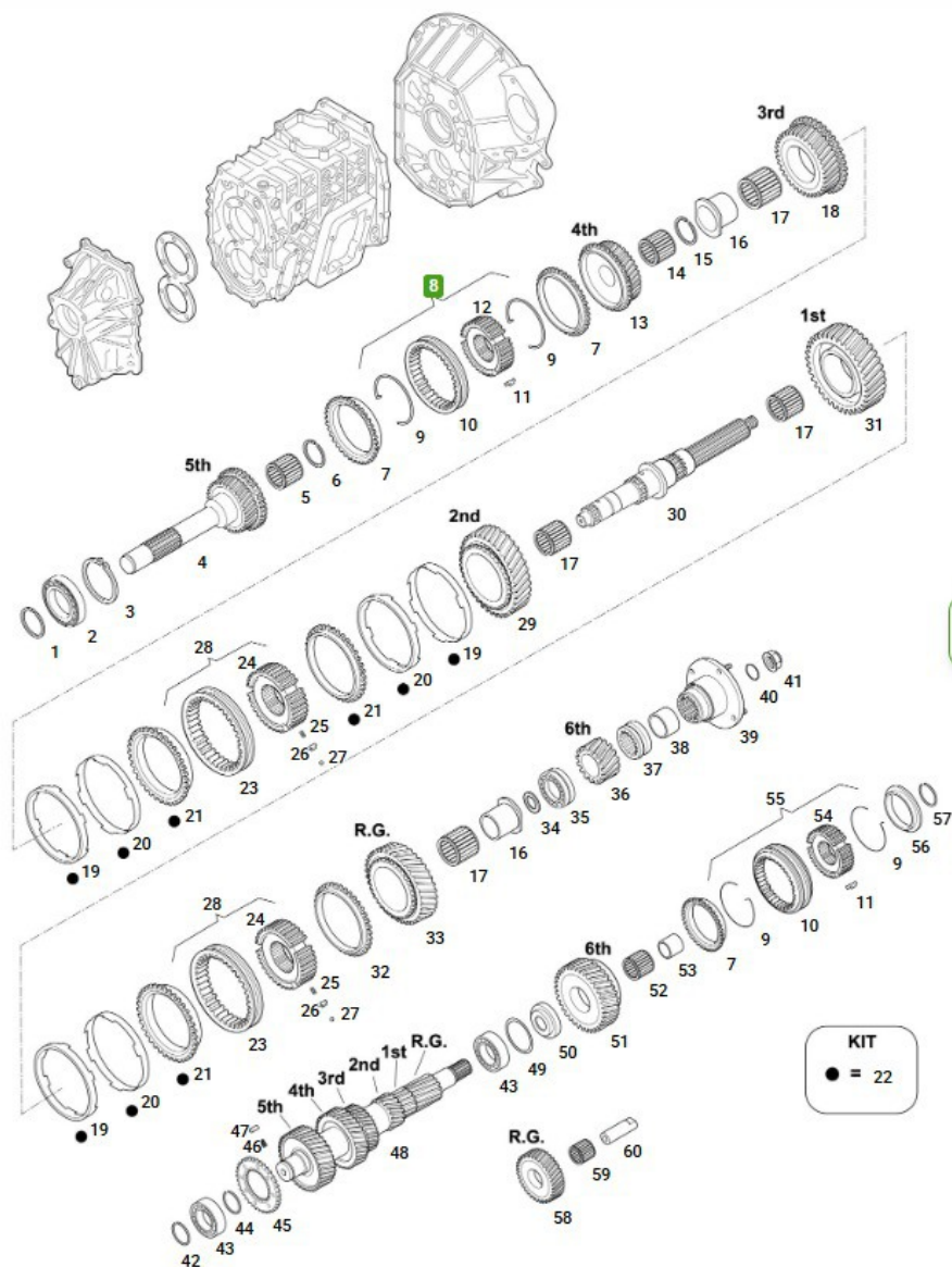
Desen tehnic cutie de viteze Isuzu MYY6S / MYY5T
