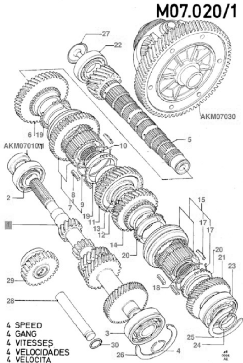
Desen tehnic cutie de viteza Ford B5, iB5
