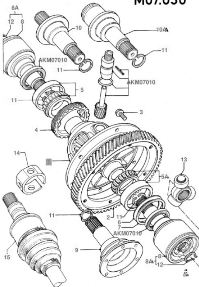
Desen tehnic cutie de viteza Ford B5, iB5
