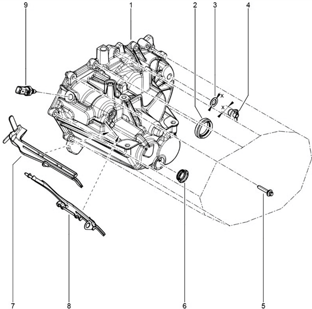
Desen tehnic cutie de viteza Dacia Dacia - JT4-023 / JT4-016 / Logan 3
