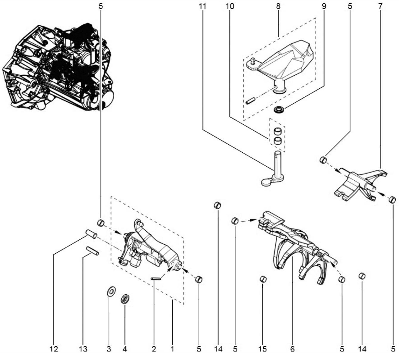
Desen tehnic cutie de viteza Dacia Dacia - JT4-023 / JT4-016 / Logan 3
