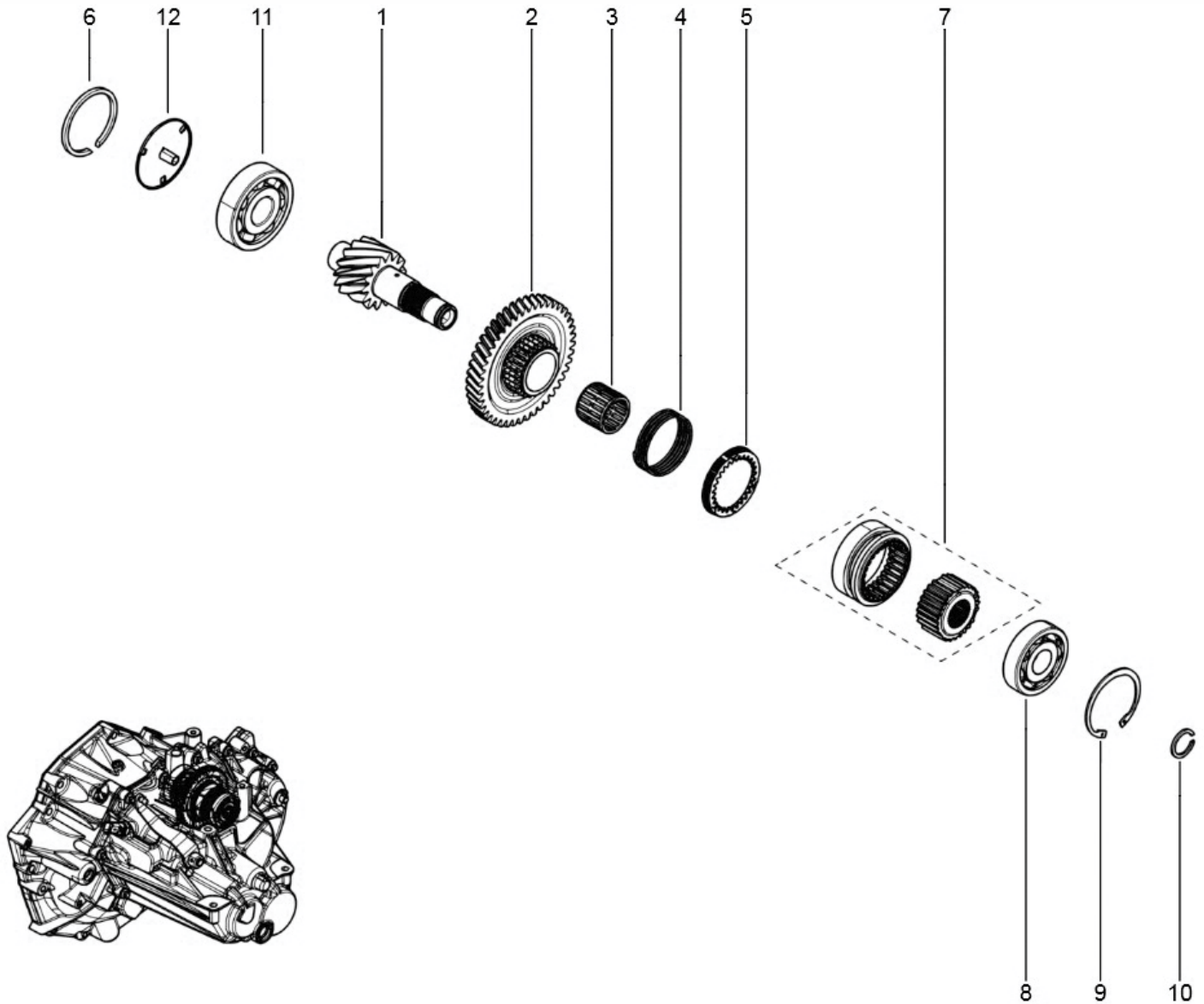
Desen tehnic cutie de viteza Dacia Dacia - JT4-023 / JT4-016 / Logan 3
