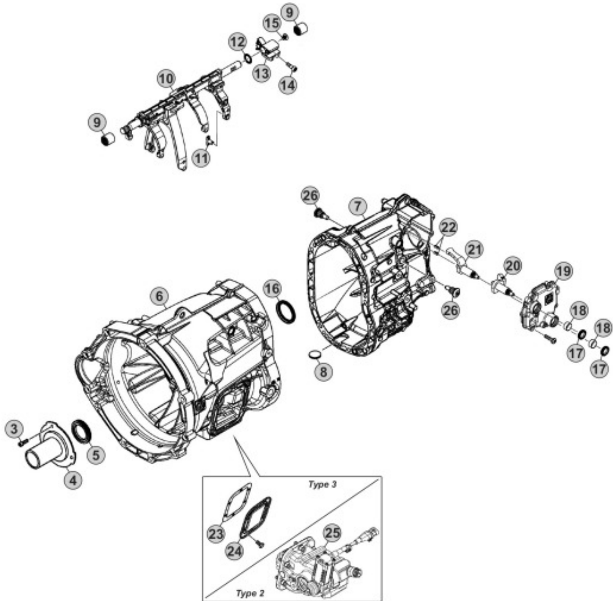
Desen tehnic cutia de viteze MAN MI410
