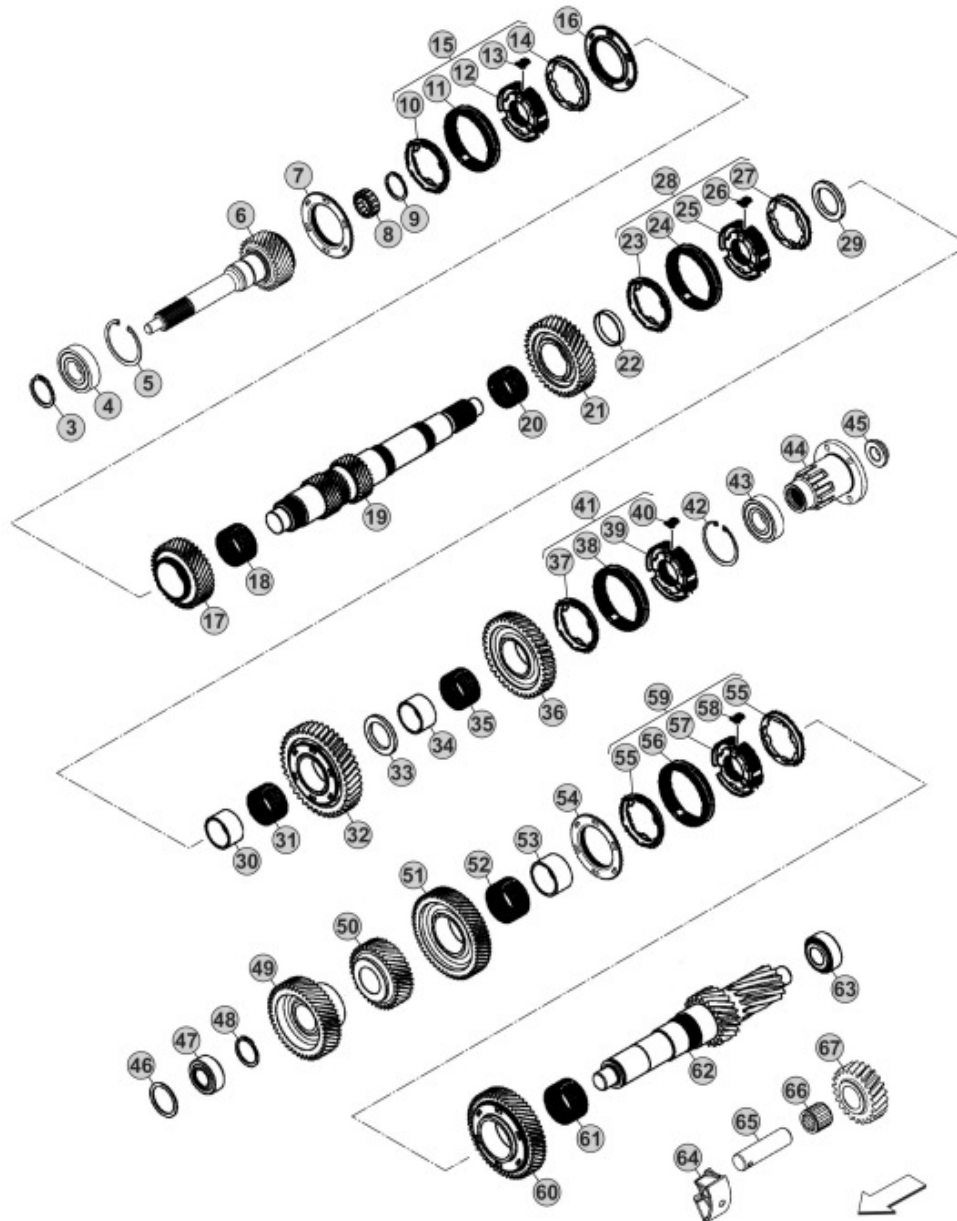
Desen tehnic cutia de viteze MAN MI410
