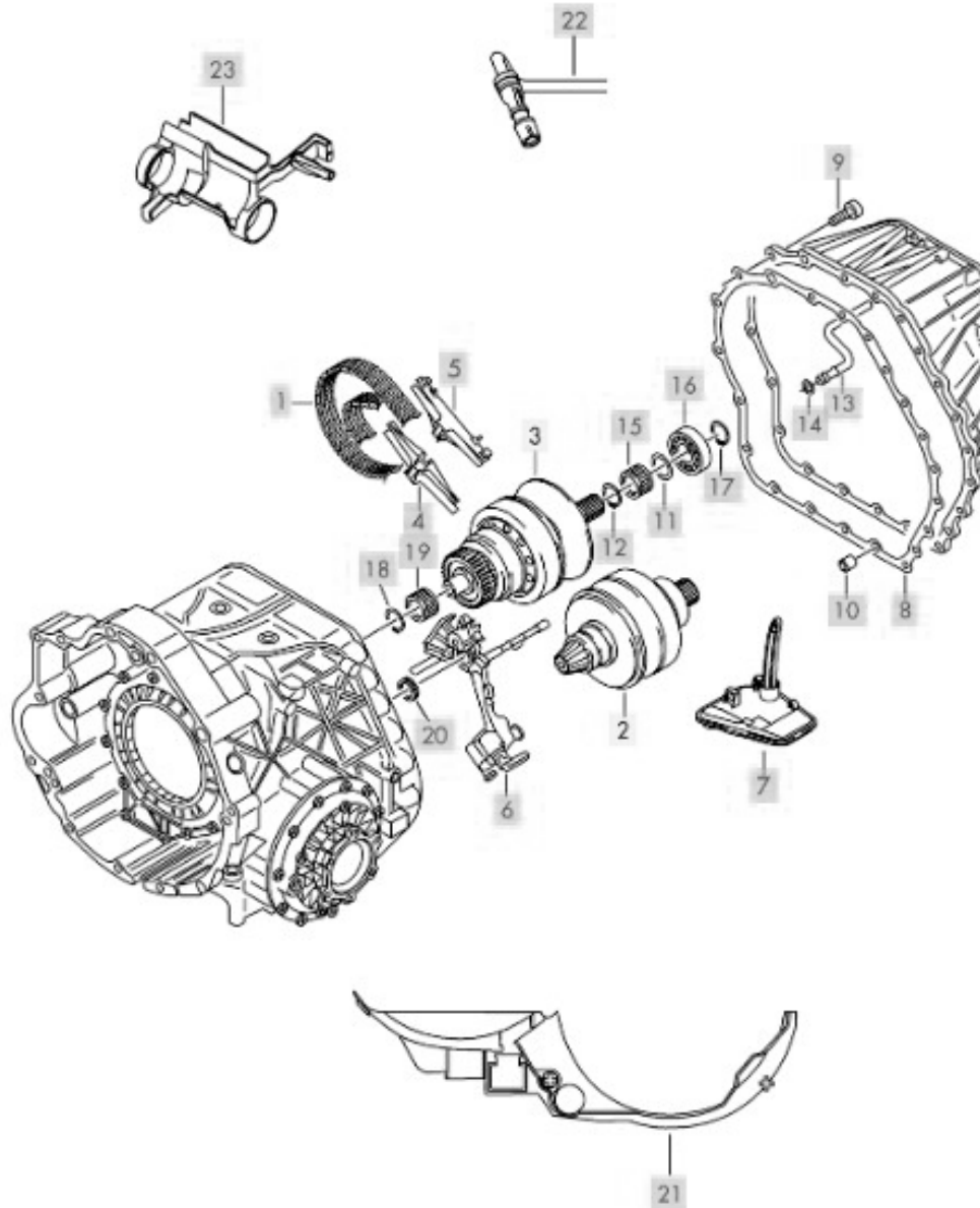
Desen tehnic cutia de viteze Audi 01J CVT Multitronic
