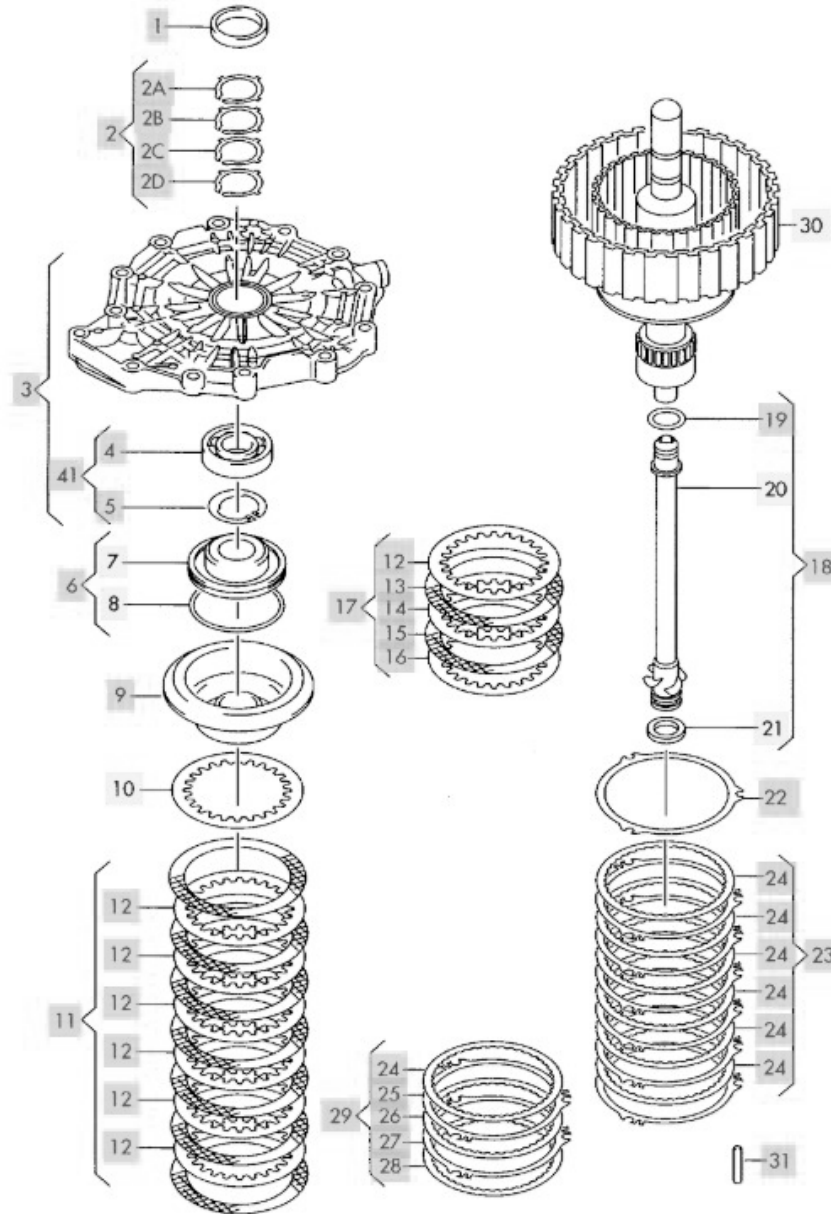
Desen tehnic cutia de viteze Audi 01J CVT Multitronic
