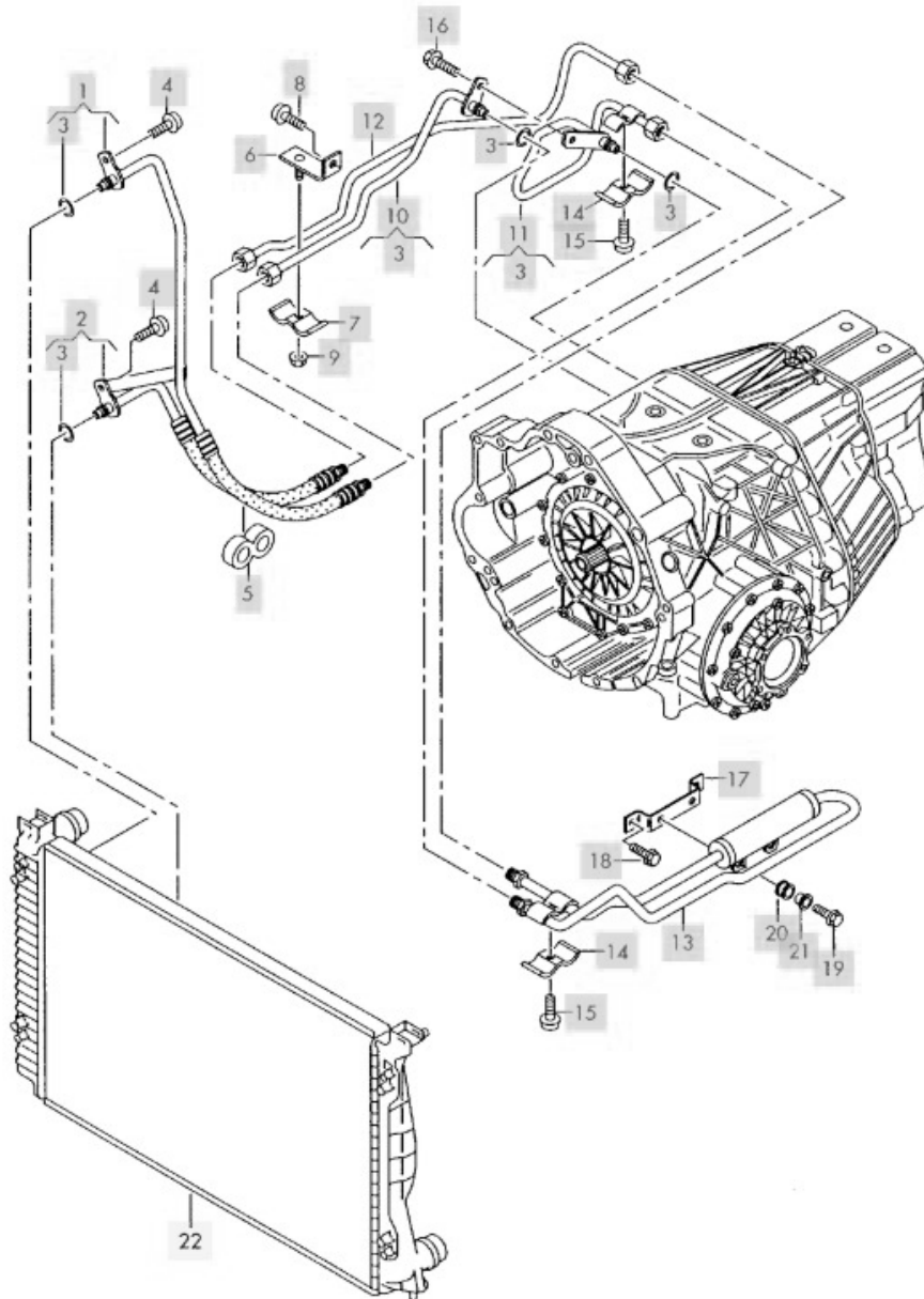
Desen tehnic cutia de viteze Audi 01J CVT Multitronic
