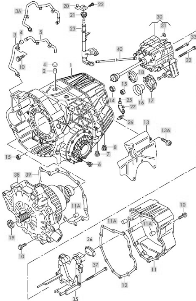
Desen tehnic cutia de viteze Audi 01J CVT Multitronic
