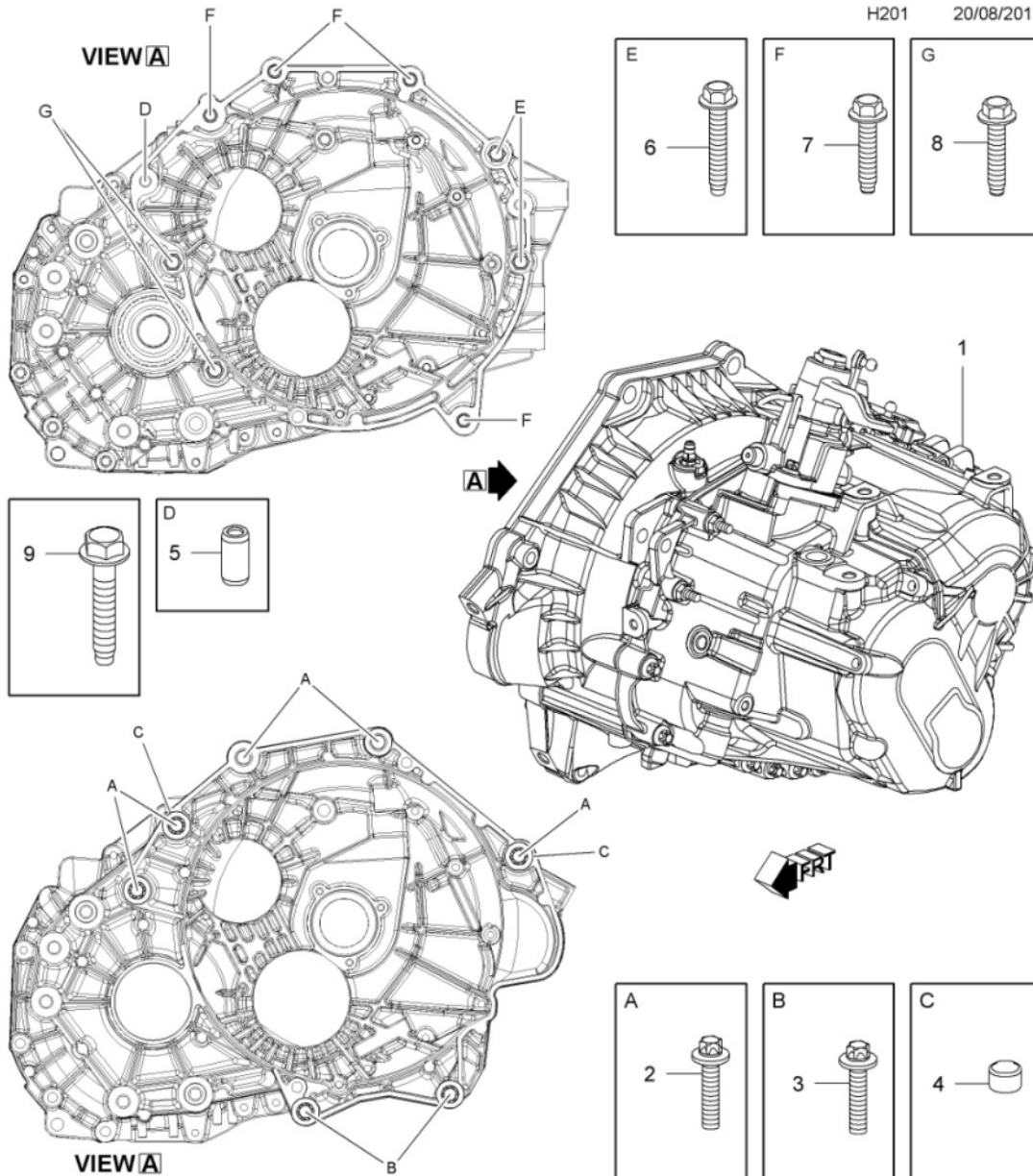
Desen tehnic cutia de viteze GM F40
