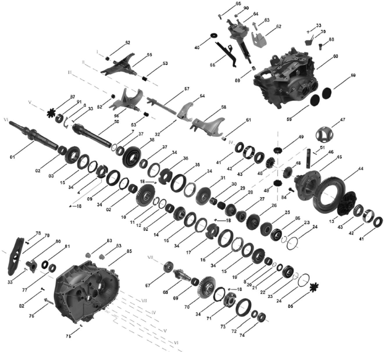
Desen tehnic cutie de viteza GS6-55BG (6sp Getrag) MINI ONE
