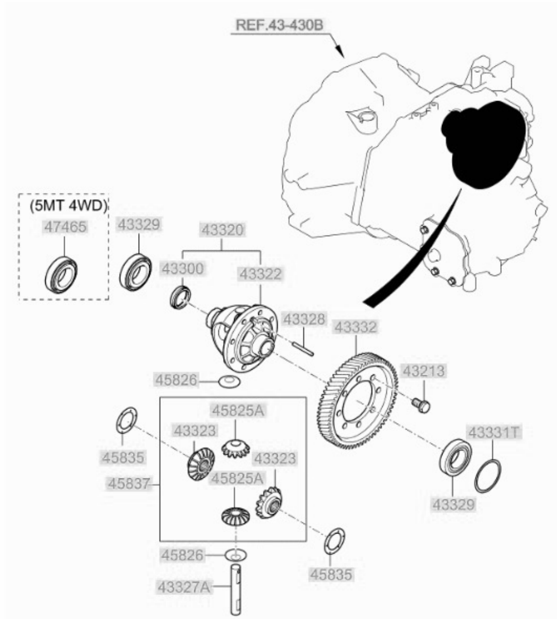
Desen tehnic cutie de viteza HYUNDAI Ix35 / TUCSON 4300039AB0
