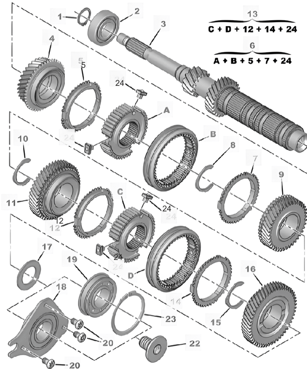
Desen tehnic cutie de viteze MC6
