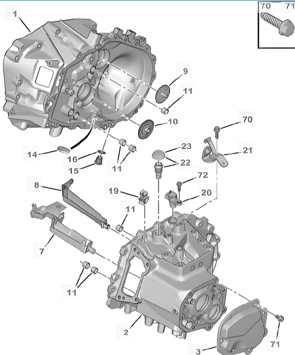
Desen tehnic cutie de viteze MC6
