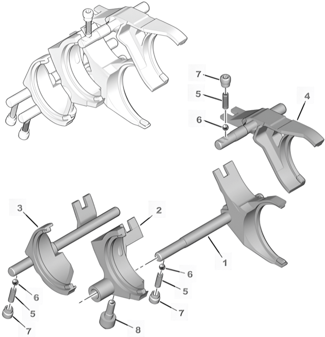
Desen tehnic cutie de viteze MC6
