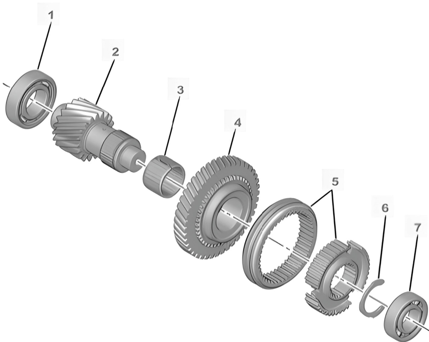
Desen tehnic cutie de viteze MC6
