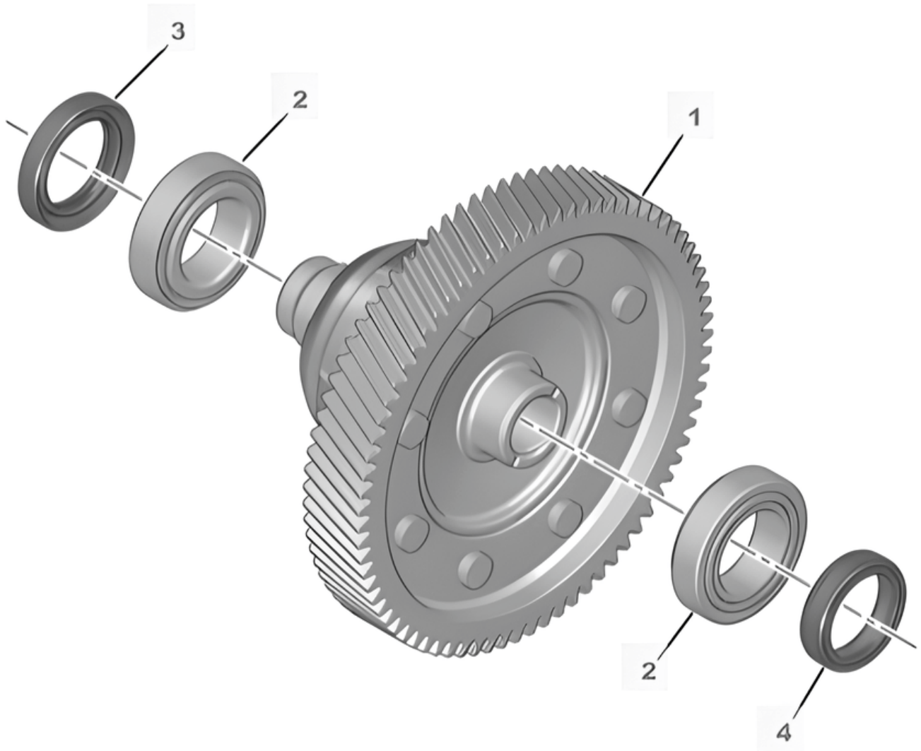
Desen tehnic cutie de viteze MC6
