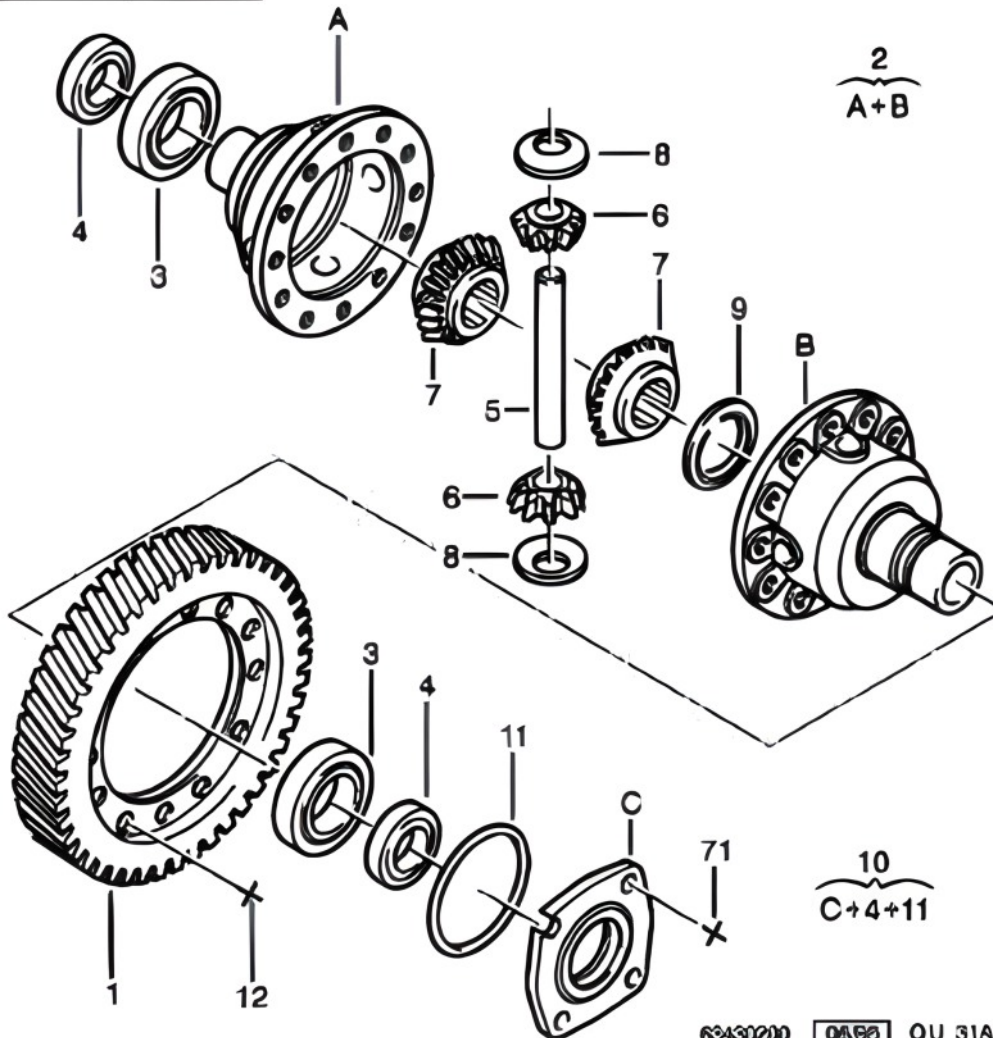
Desen tehnic cutie de viteza ME5K, C504
