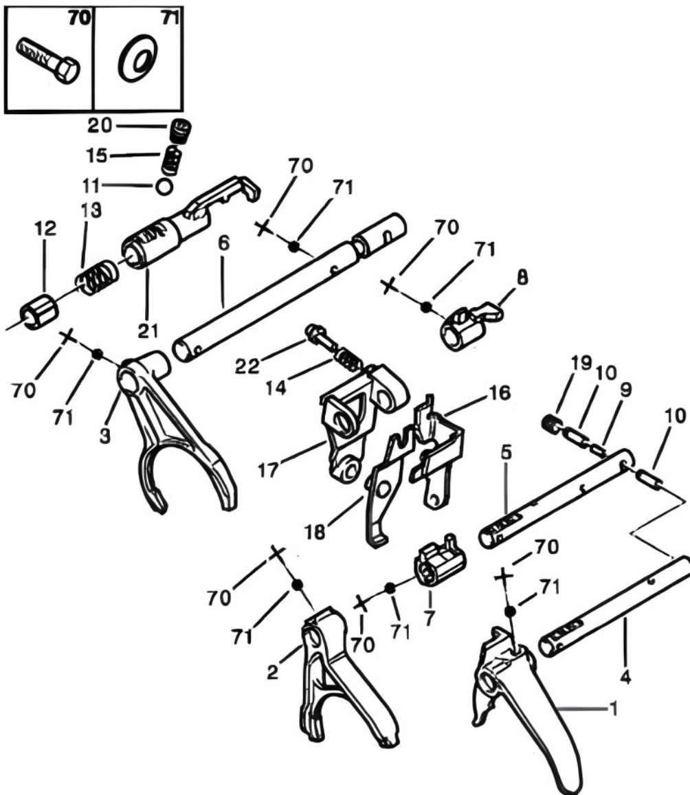
Desen tehnic cutie de viteza ME5K, C504
