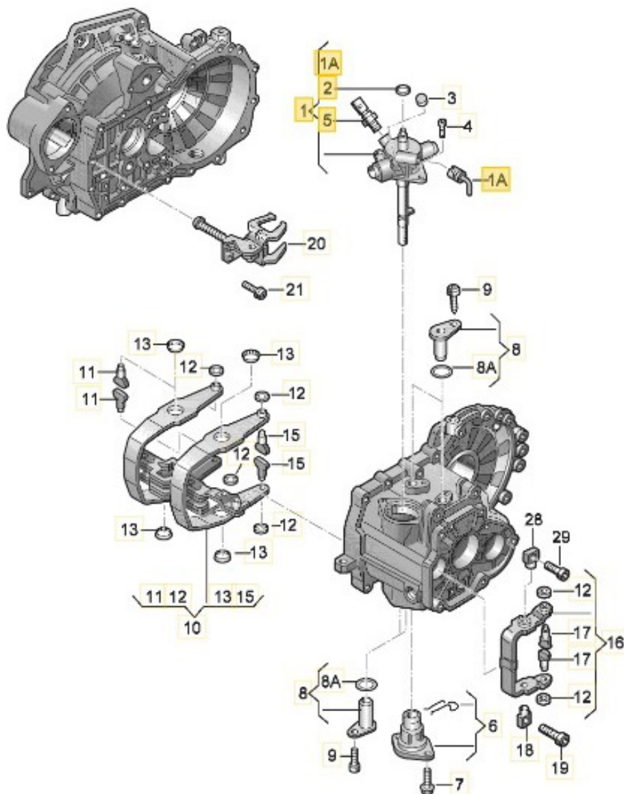
Desen tehnic cutie de viteza 02A 02J 0A4 02R 02S (5 & 6 speed)
