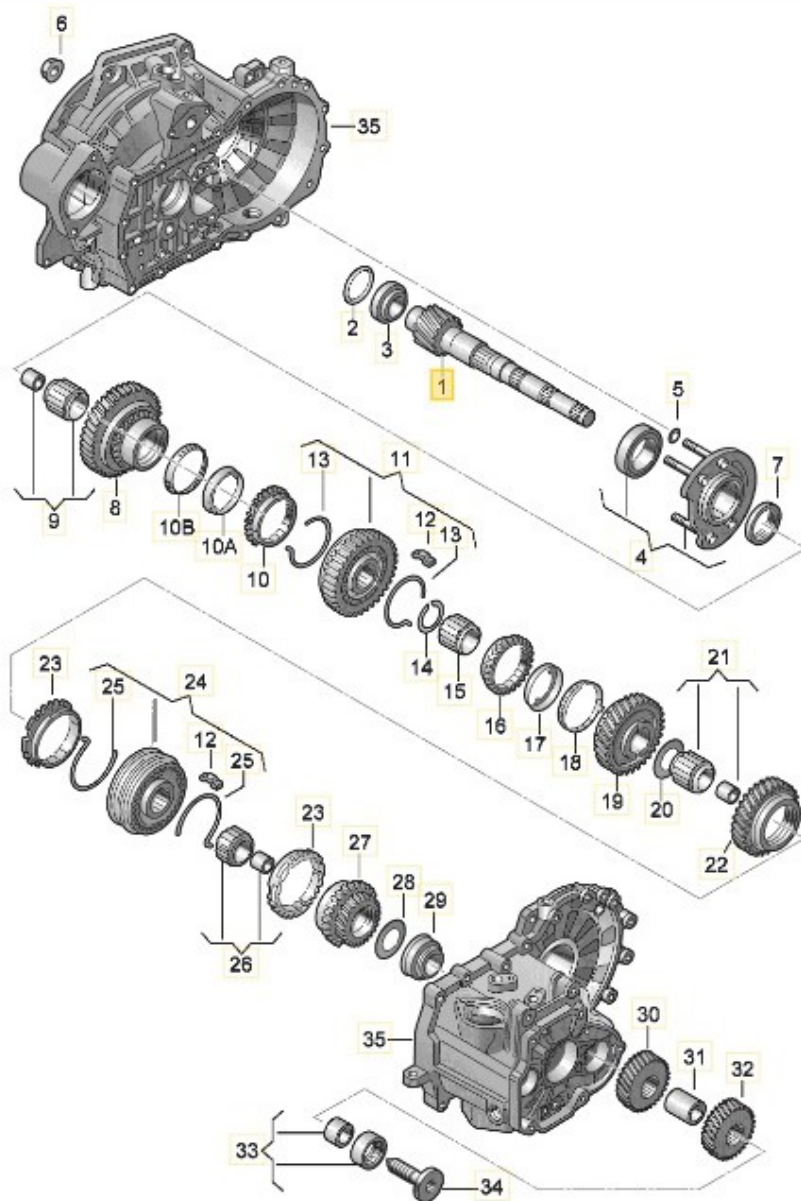
Desen tehnic cutie de viteza 02A 02J 0A4 02R 02S (5 & 6 speed)
