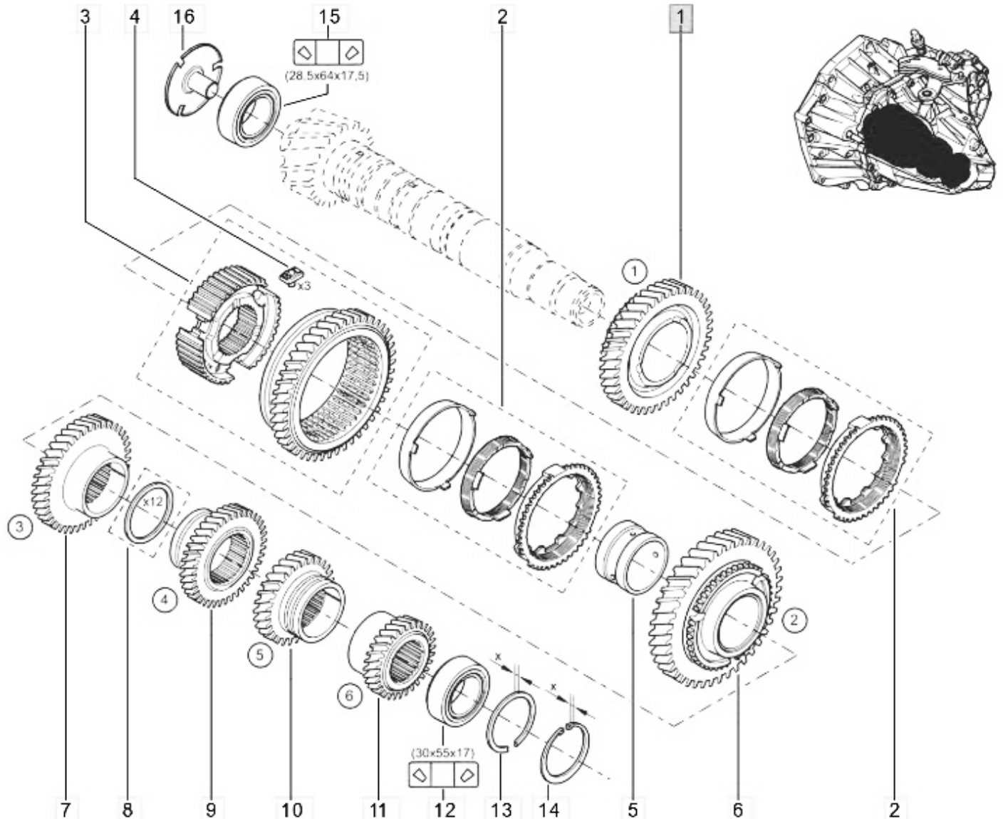
Desen tehnic cutie de viteza Dacia Duster - TI8
