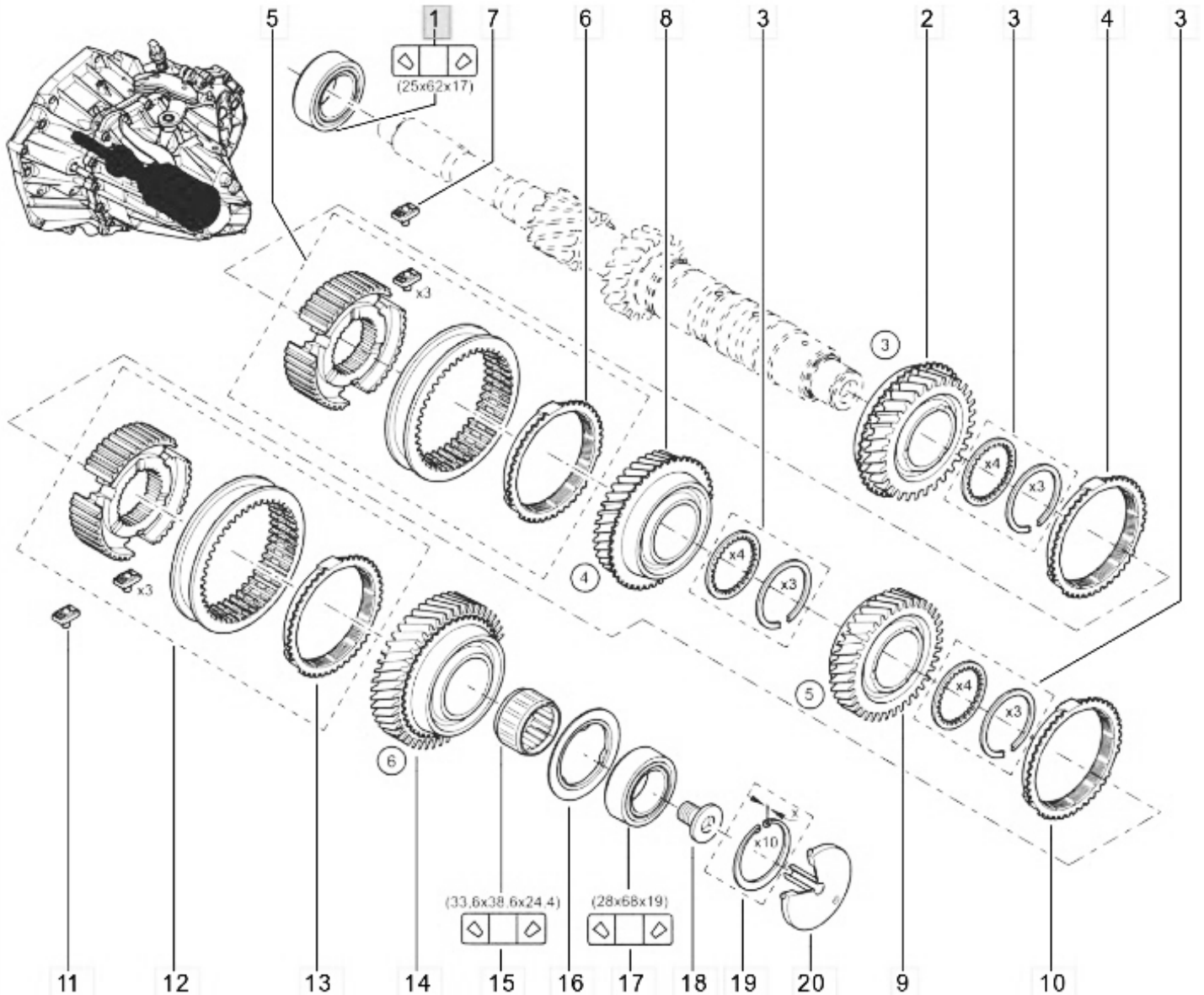
Desen tehnic cutie de viteza Dacia Duster - T18
