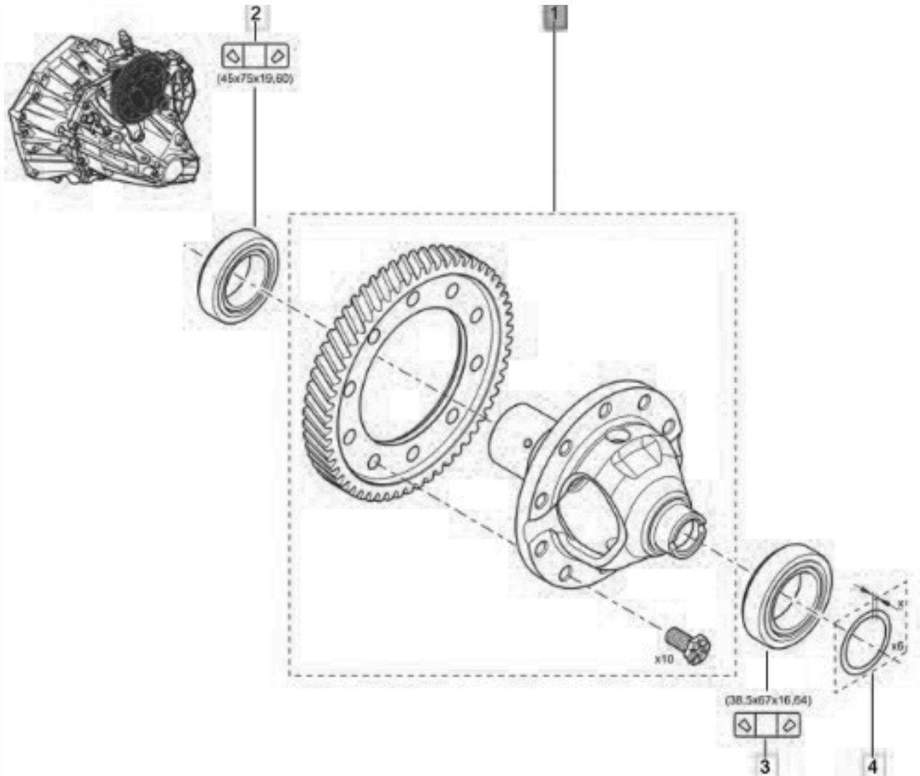
Desen tehnic cutie de viteza Dacia Duster - T18
