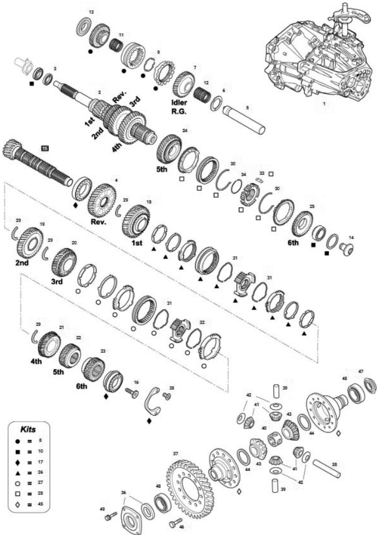
Cutia de viteza ML6 - Fiat / Citroen / Peugeot
