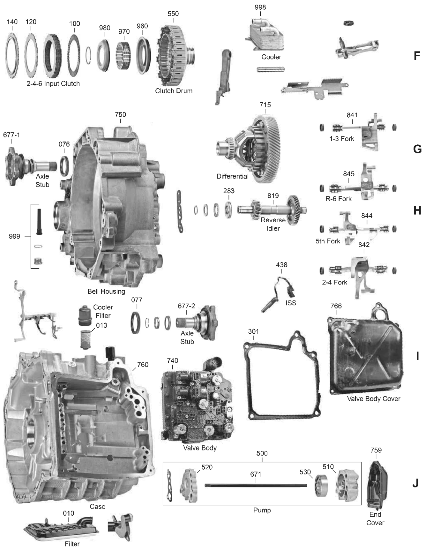
Desen tehnic cutie de viteza DQ250 - 6 TREPTE
