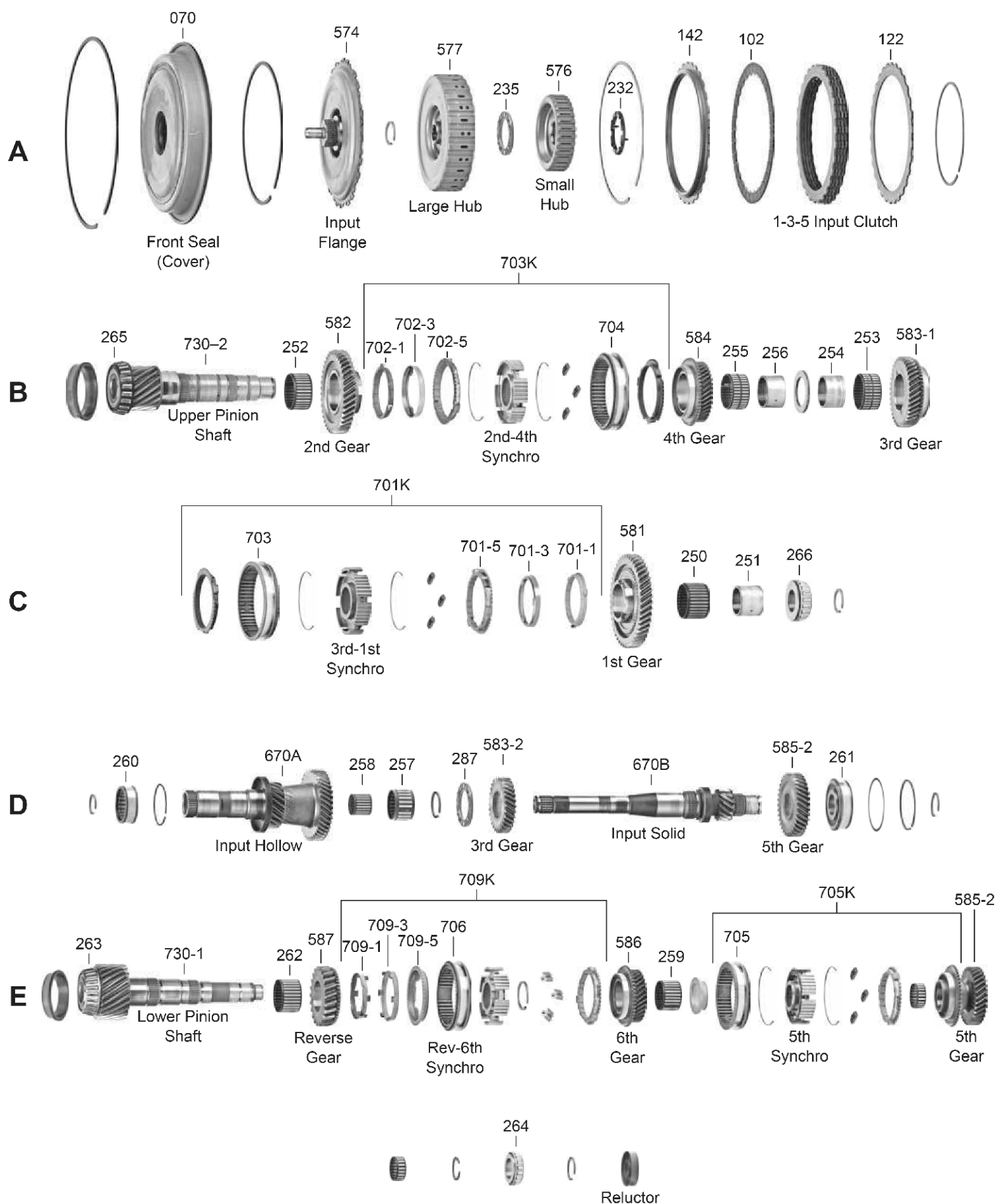
Desen tehnic cutie de viteza DQ250 - 6 TREPTE
