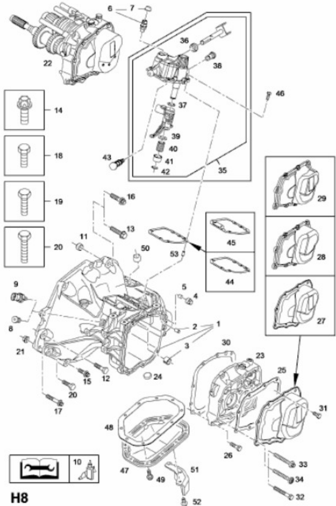
Desen tehnic cutie manuala F17
